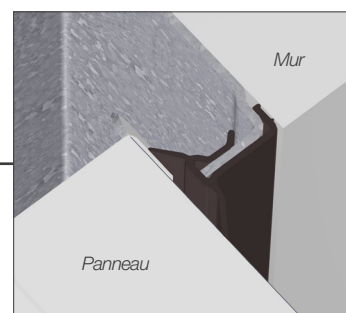
Joint à lèvres (sur rails verticaux)
