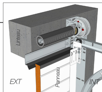
Vue extérieure Joint avec 2 lèvres
