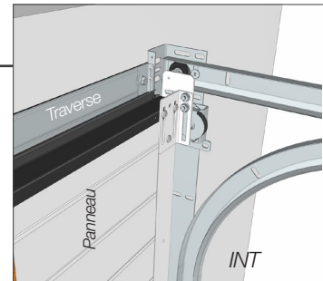
Vue intérieure Joint avec 2 lèvres (linteau)
