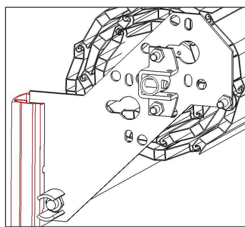
Flasque positionnée dans la Coulisse
