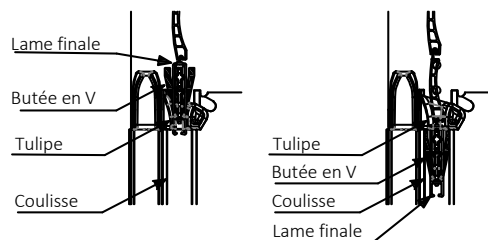
Lame finale
