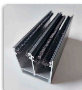
Coulisses C48T Coulisse double avec joint brosse
