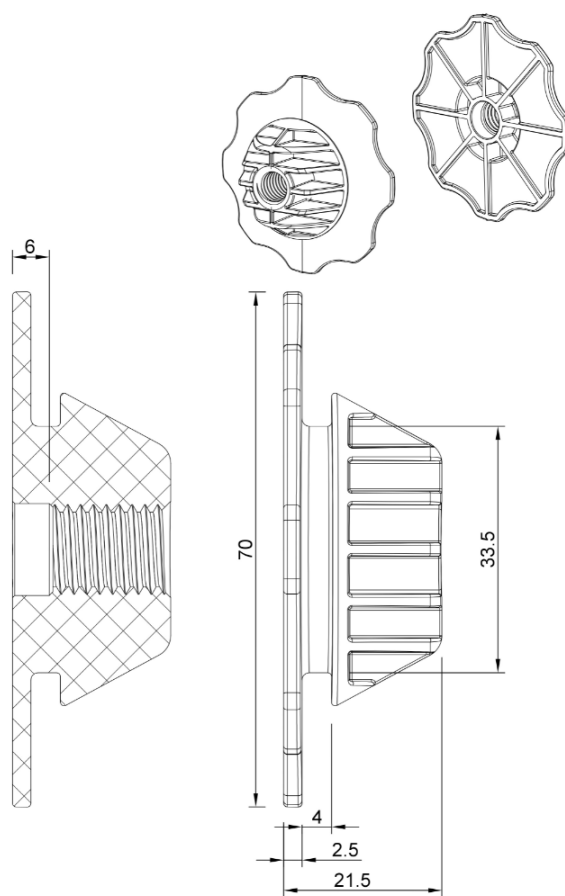
Figure 17 - Connecteur
