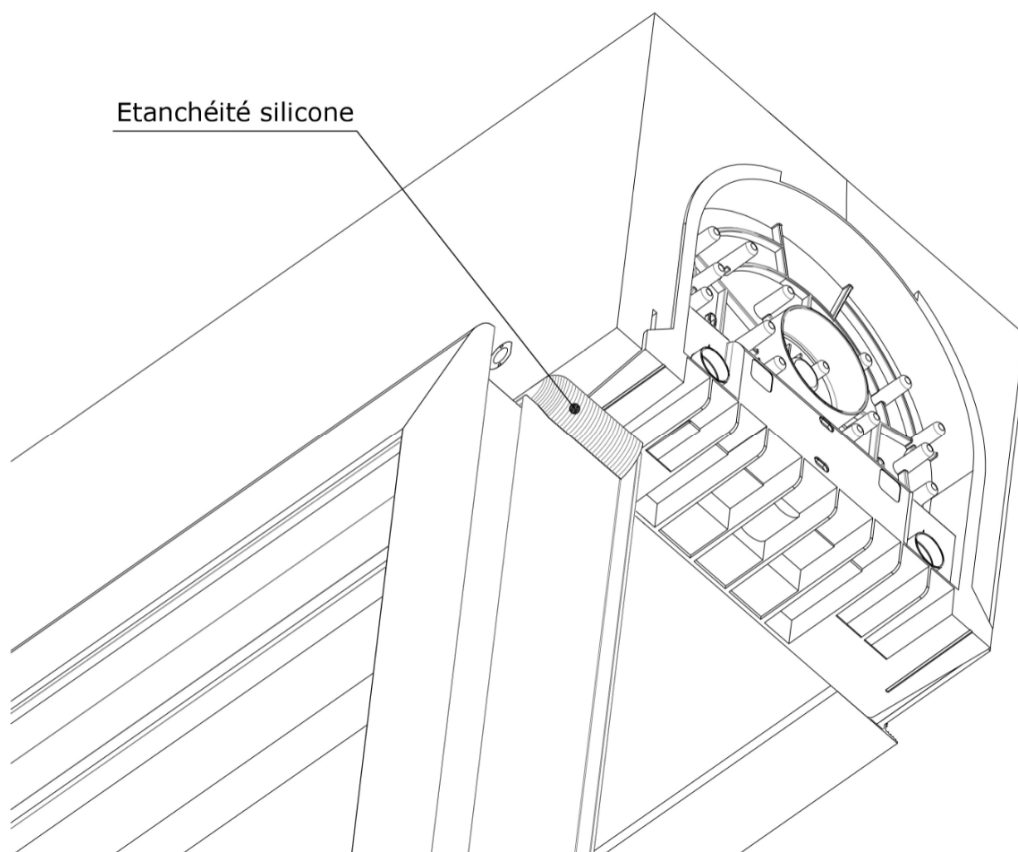
Figure 30 – Etanchéité Joue/Menuiserie
