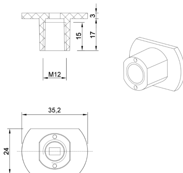
Figure 17 - Connecteur
