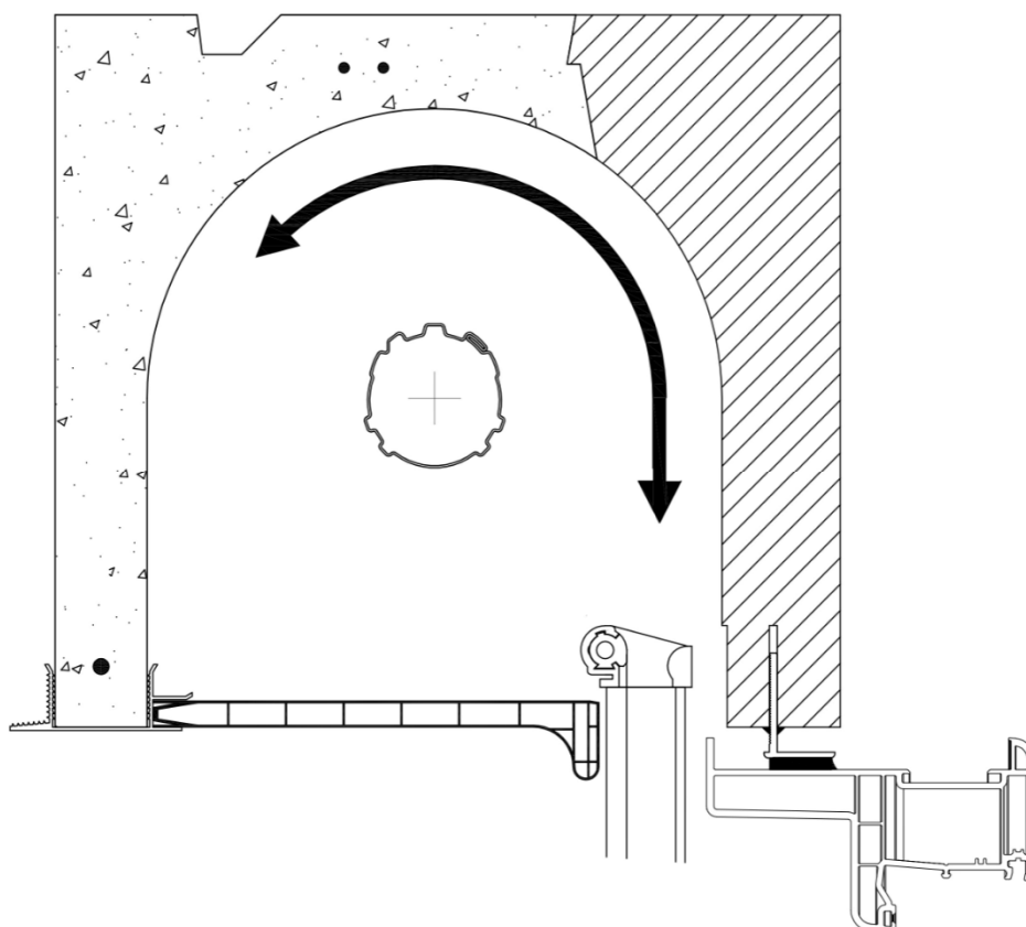
Figure 6 - Enroulement intérieur
