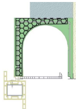
Renfort interne + rail PVC à languette
