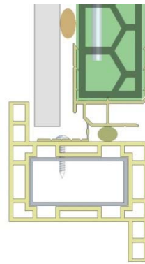
Avec le rail PVC à languette
