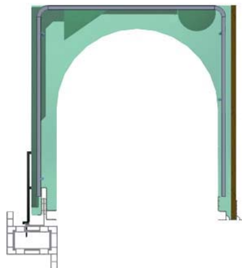
Renfort interne + rail PVC à languette
