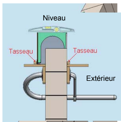
Alignement nu extérieur
