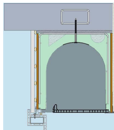
Fixation du tirefond en pose dans réservation ou sous dalle
