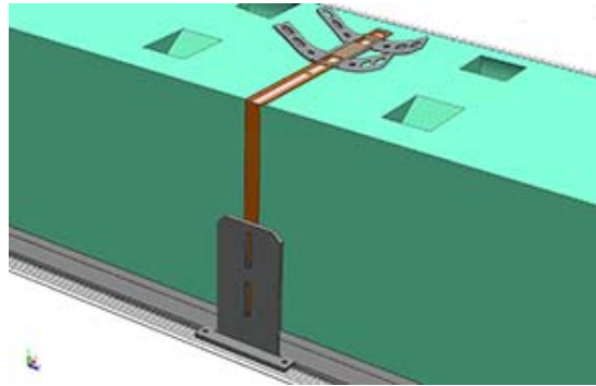
Relever les 'ailes' du renfort N°5 pour les sceller dans le linteau
