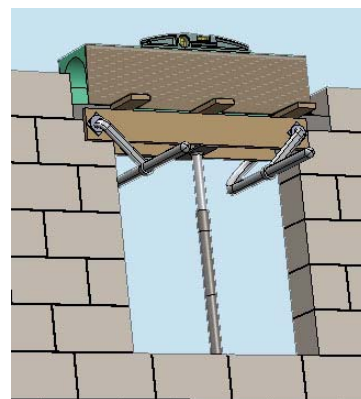
Échafaudage et mise à niveau
