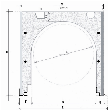
La prise de côtes
