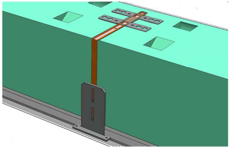
Visser le renfort N°4
