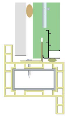
Avec le rail Télescopique mono paroi
